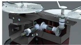
Prevodovka v olejovej náplni
