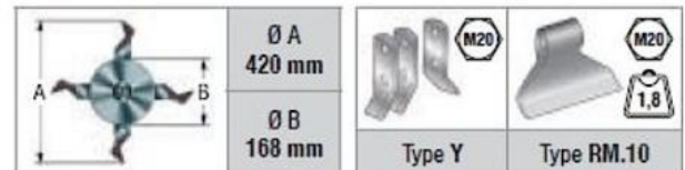
Priemer rotora a vlastnosti kladív
