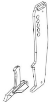
Podryvacia radlička GLS
